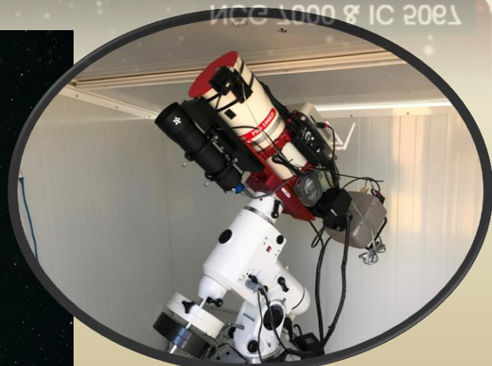
NCG 7000 & IC 5067
